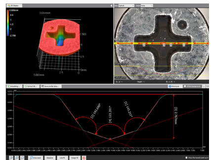
十字螺絲頭內角度測量
